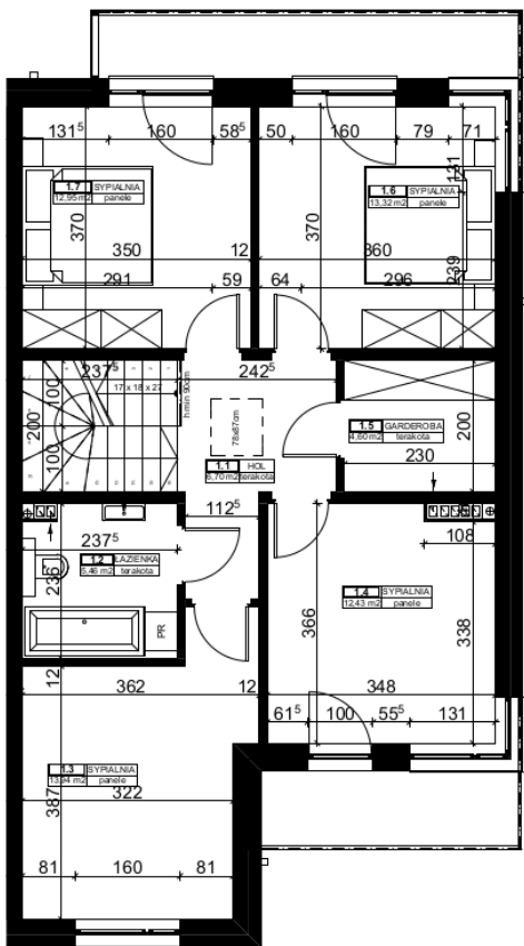
piętro
