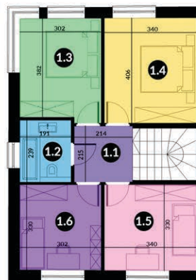
I piętro
