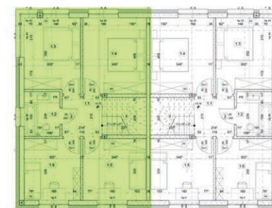
II piętro
