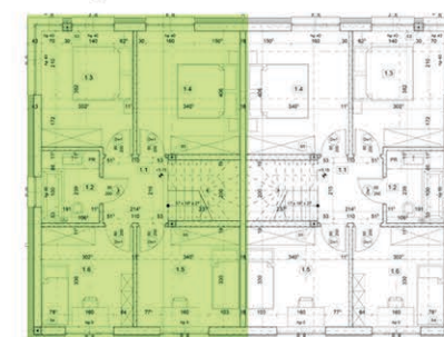
I piętro
