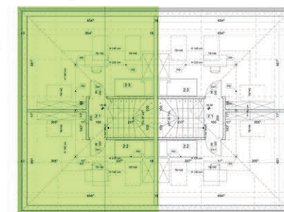
II piętro
