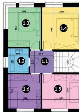
I piętro
