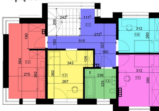
I piętro
